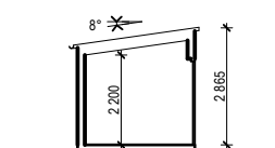
SEKTION A-A
